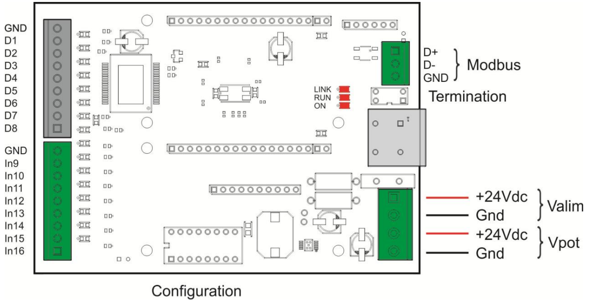
Fig.: ModBus Serial port
