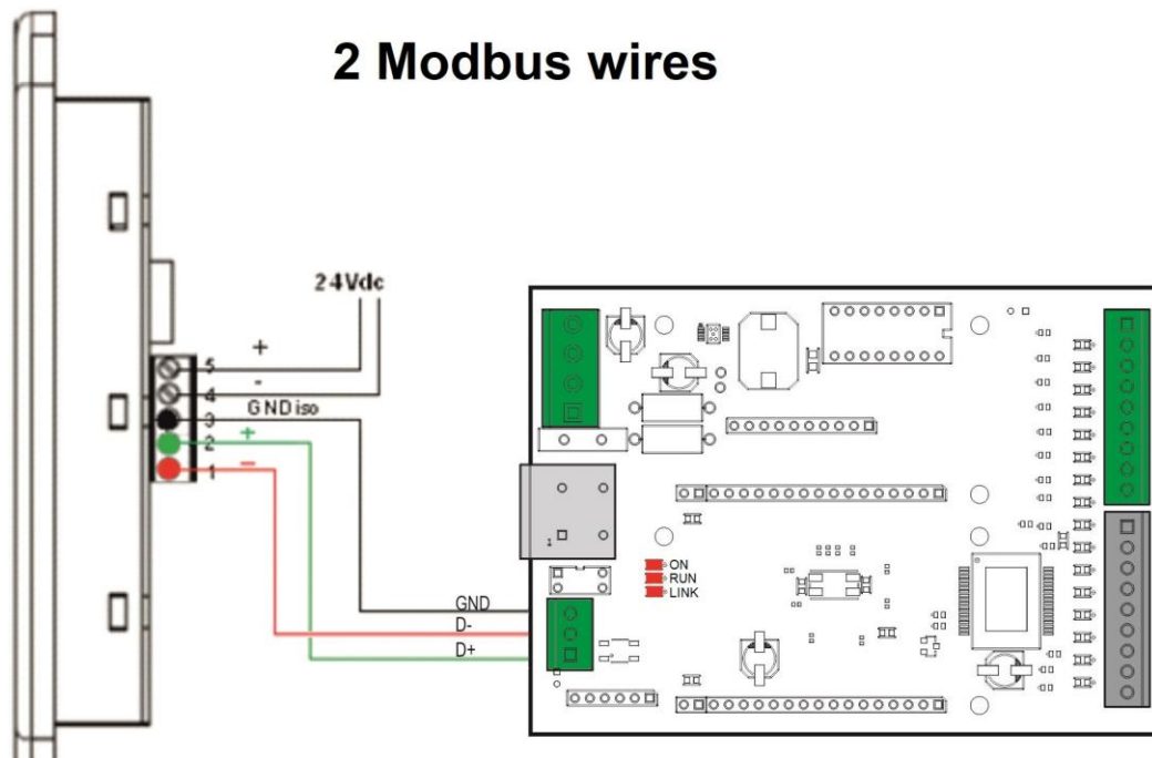
Fig.: Modbus connection
