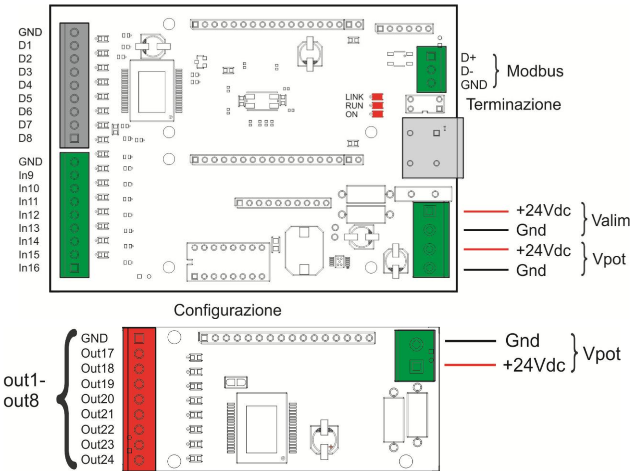
Fig.: Collegamenti uscite digitali
