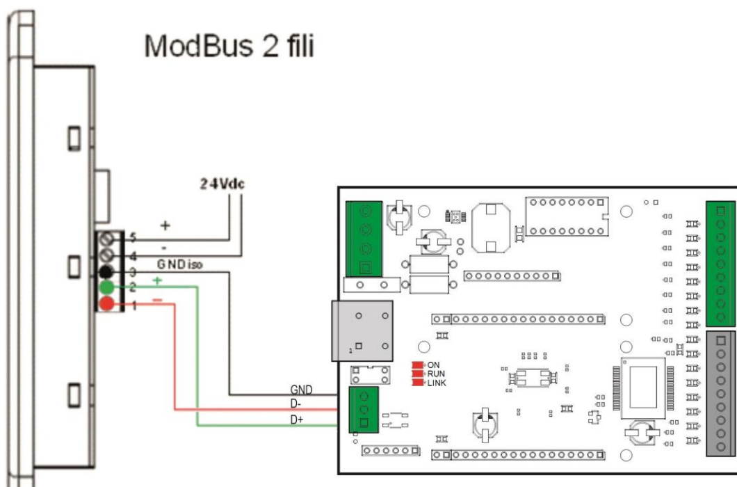
Fig.: Collegamento Modbus
