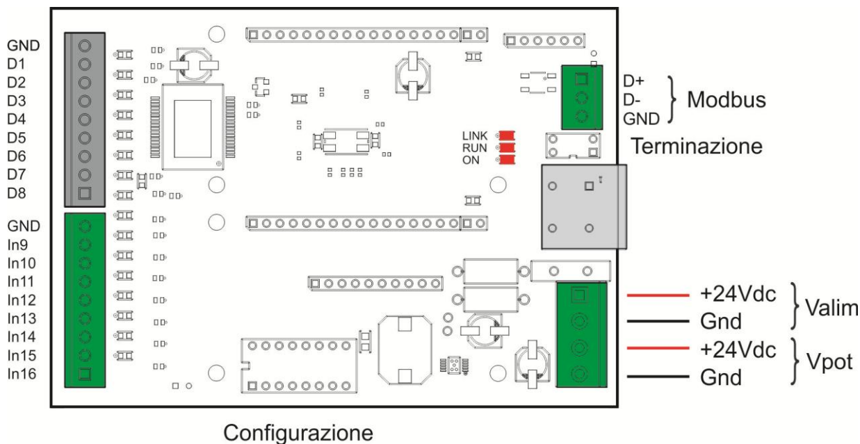
Fig.: Seriale ModBus
