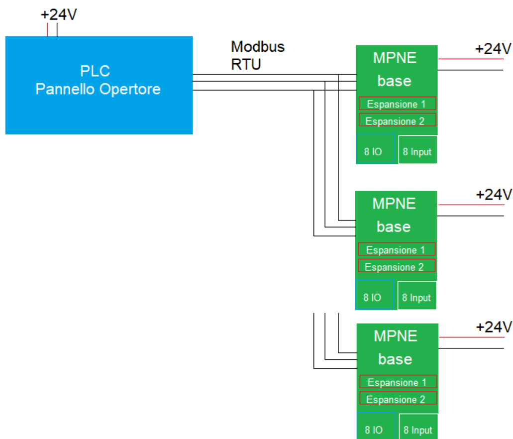
Fig.: catena logica
