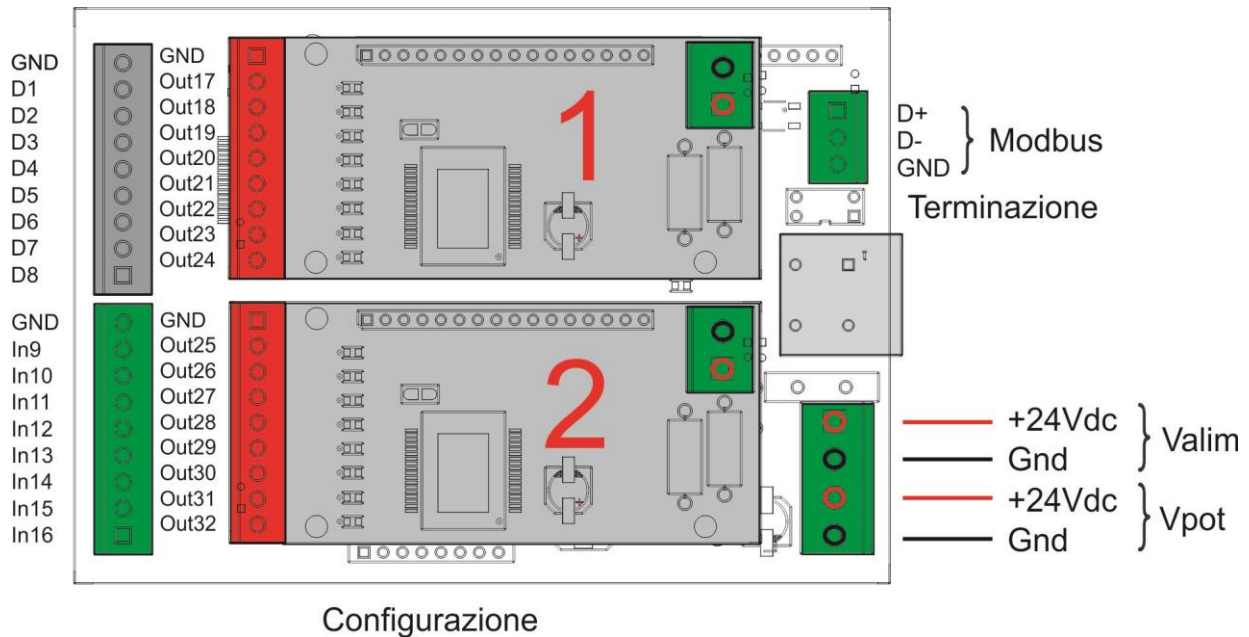
Fig.: Collegamenti Base + uscite digitali (schede Espanse)
