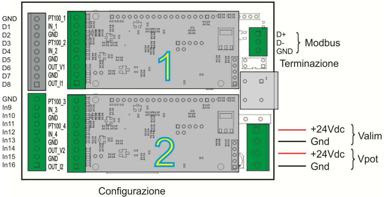
Fig.: Collegamenti Base + ingressi /uscite analogici (schede Espanse)
