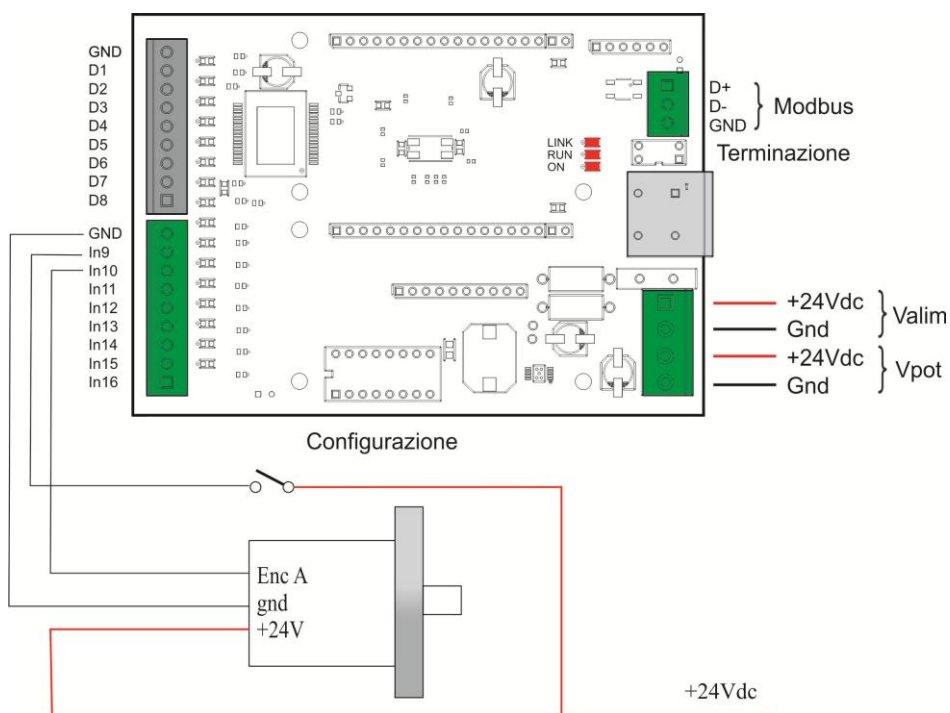
Fig.: Collegamento encoder monodirezionale
