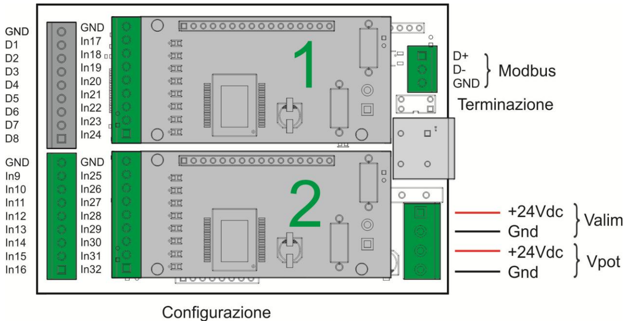
Fig.: Collegamenti Base + ingressi digitali (schede Espanse)
