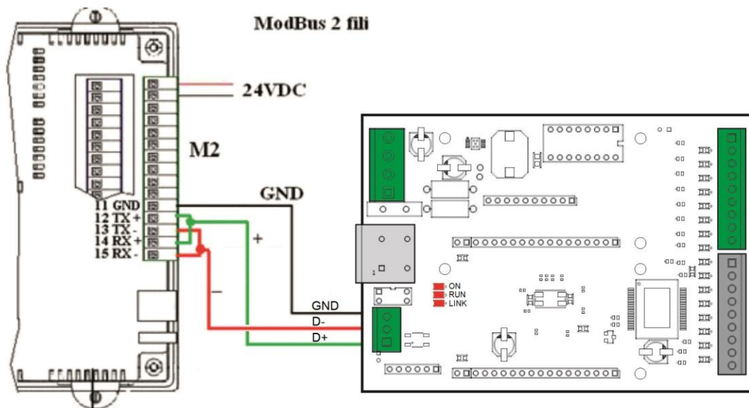
Fig.: Collegamento Modbus
