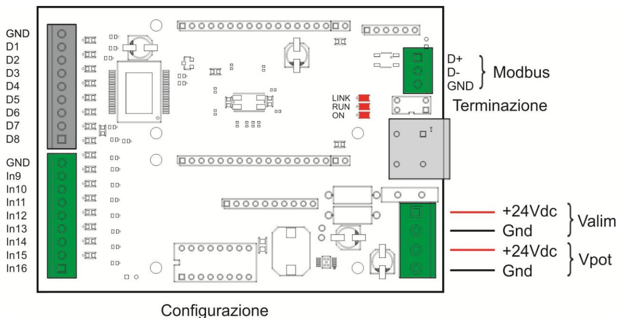
Fig.: Collegamenti Base
